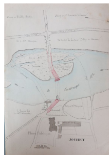
Plan pour l'amélioration des rampes d'accès au bac de Jouhet, avec mention du gué, du bac et du barrage de l'ancien moulin, par Delafont ingénieur, 1857
