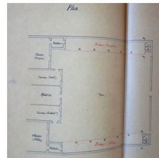
Construction de préaux et réparations au groupe scolaire. Plan et coupes des ouvrages, par Plat architecte, 1912.
